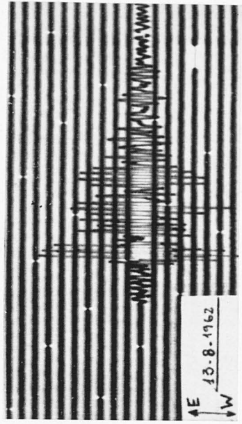
Fig. 25 - Comp. E-W di una scossa avvenuta nei pressi di Tolmezzo (13-VIII-1962), e registrata a Pieve di Cadore, alla distanza di 55 km ca.
