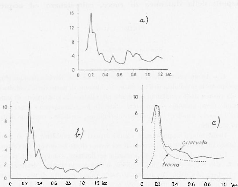
Fig. 1 — a) Rapporto ampiezze osservate in superficie e a 300 m di profondità nella miniera di Hitachi (Giappone);
