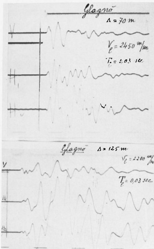
Fig. 5 - RegISTRAZIONI vibrografiche in roccia poco compatta, a basso modulo di elasticità (il periodo delle onde sismiche è notevolmente più alto di quello delle oscillazioni, di cui alla fig. 4).
