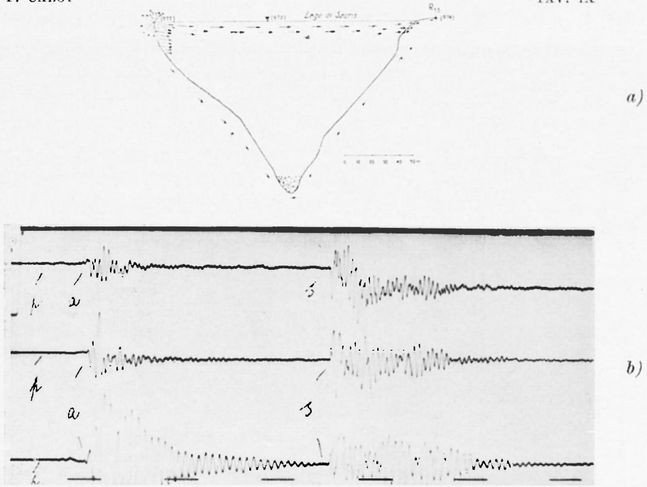
Fig. 14 - a) Scoppio in S_{13} , registrazione in R_{12} , sull'altra sponda del lago; b) onde p trascurabili, ampie le a che hanno attraversato l'elemento liquido.
