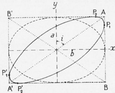
Fig. 36 - Composizione di moti armonici a 90°.
