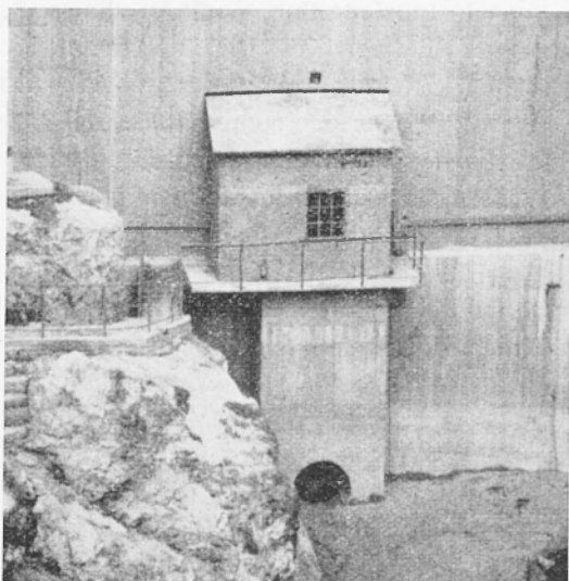
Fig. 28 bis - Diga dell'Ambiesta: casetta-custodia dei clinografi diga (q. 437,5) e tampone.
